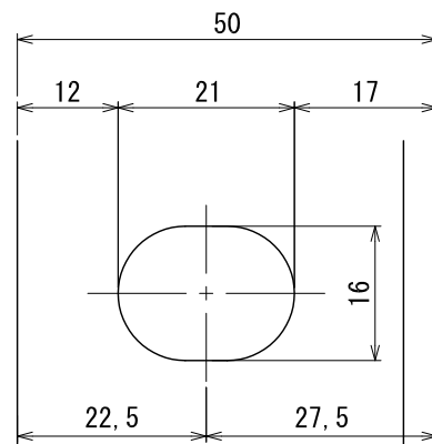
<長穴 拡大図>
