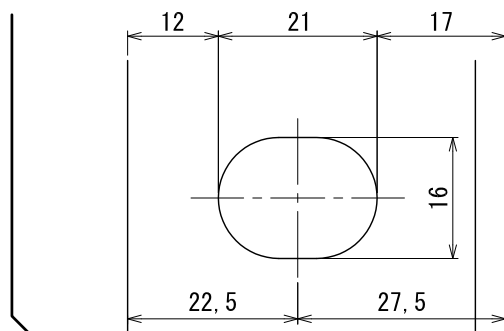
<長穴 拡大図>
