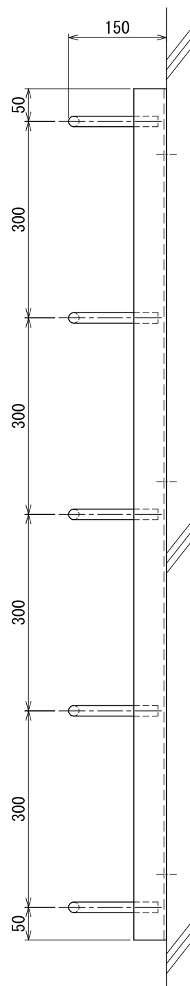
<長穴 拡大図>
