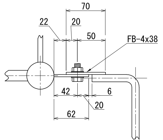
《ガード取付部詳細図》
