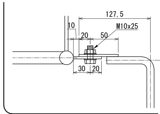
ガード取付部詳細図
