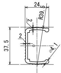
支柱形状
