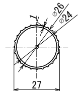
ステップ形状
