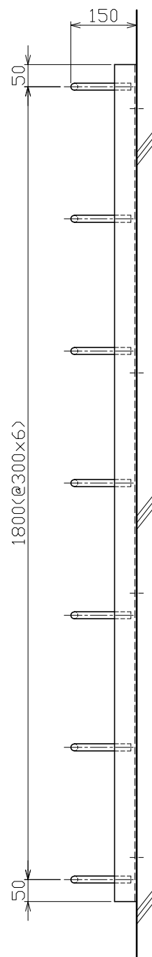
< 長穴 拡大図 >
