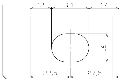
< 長穴 拡大図 >
