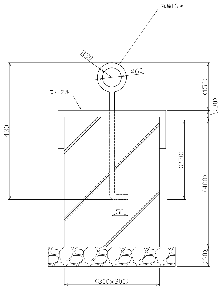
下端金物（独立の場合） C082B
