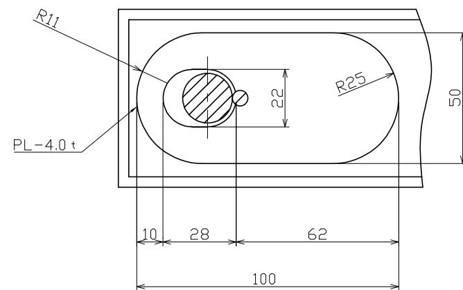
スライド板詳細図
