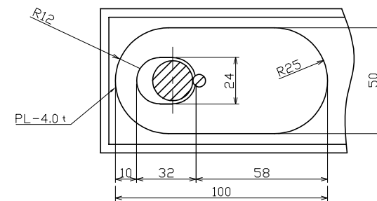
スライド板詳細図
